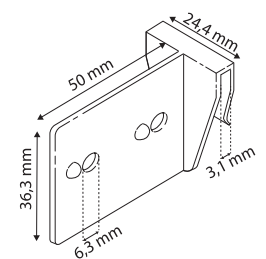
Plastični dodatak za fiksiranje na police ili panele 3,1 mm max debljine i ojačavanje kartonskih polica. Dužina 24,4 mm i veličina ekstenzije 50x36,3 mm. Ima dve rupe 6,3 mm na koje se može staviti print, razdaljina između rupa 25,4 mm. Boja: bela.
